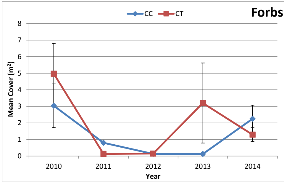
e. Forbs, Chilili.
